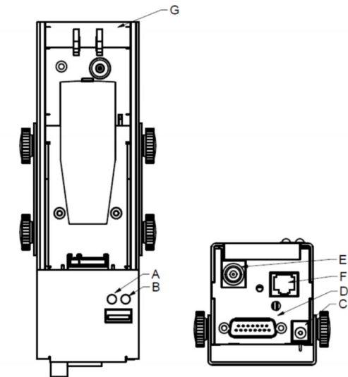
Schemazeichnung WTC1712
